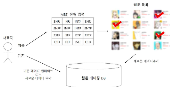
Fig. 4. 레이팅 데이터 수집 방법
