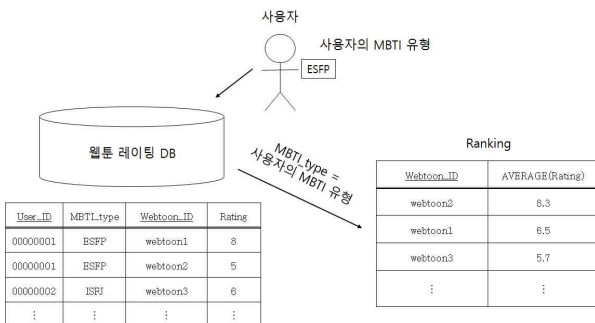
Fig. 2. 웹툰 레이팅 데이터베이스를 이용하여 추천하는 방법
